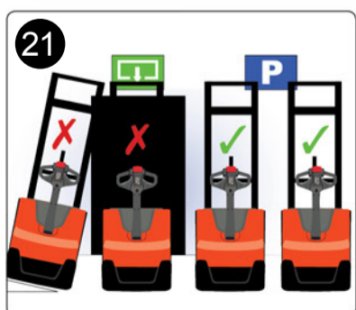
21 Stellen Sie Geräte immer in den dafür vorgesehenen Bereichen ab, lassen Sie das Gerät niemals unbeaufsichtigt. Niemals auf Rampen parken
