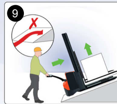
9 Beim Bergauffahren langsam und mit gehobener Last fahren, immer in Richtung Anstieg. Niemals am Anstieg wenden!
